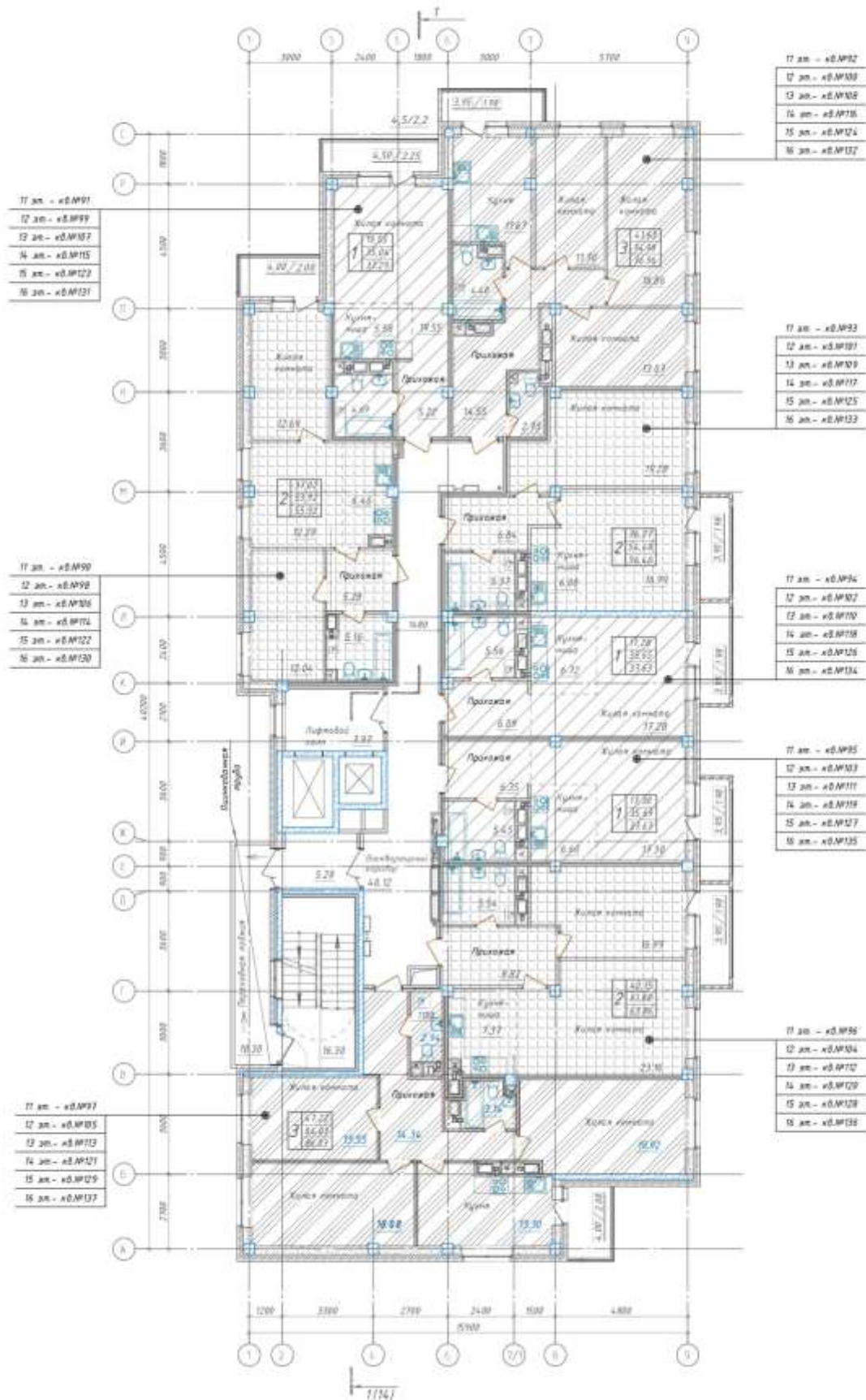
Схема плана типового этажа (11-16 эт.) с нумерацией квартир
